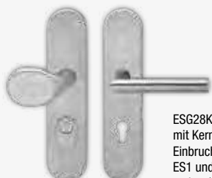
ESGR28K 670 PZ 72 mm mit Kernziehschutz rechts / links verwendbar
